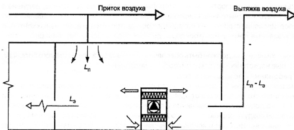
Рисунок 2 - Применение автономного устройства очистки воздуха в помещениях групп 3 и 4
